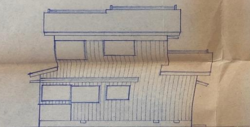
西立面图
