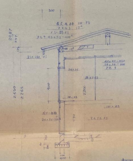
車庫矩計圖
