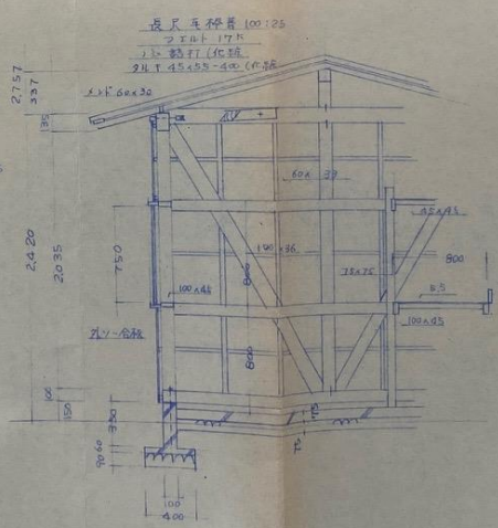
倉庫矩計圖
